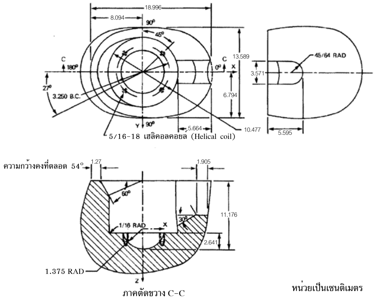
รูปที่ ข.2 คีระหัดสอบขนาดกลาง (ข้อ 4.1.2 และข้อ 10.4.1.2)
